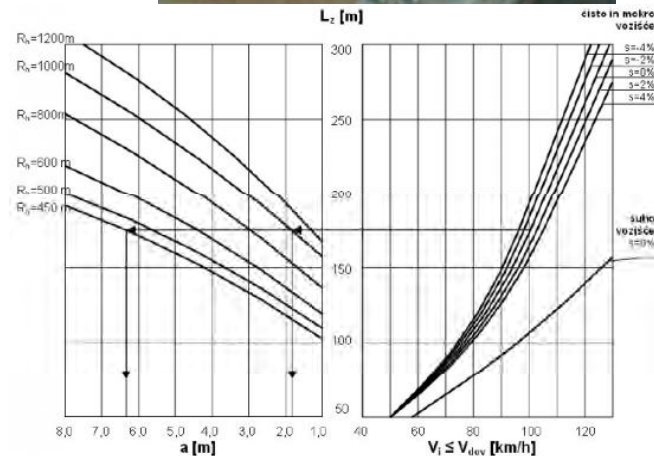
Slika III-2: Soodvisnost polmera R_0 , razdalje a , hitrosti V_1 in nagiba nivelete s (povzeto po: RAS-L, 1995)
